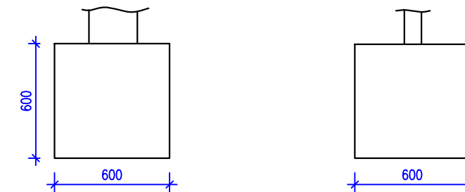
Вариант 1 (фундамент 600х600х600мм)
